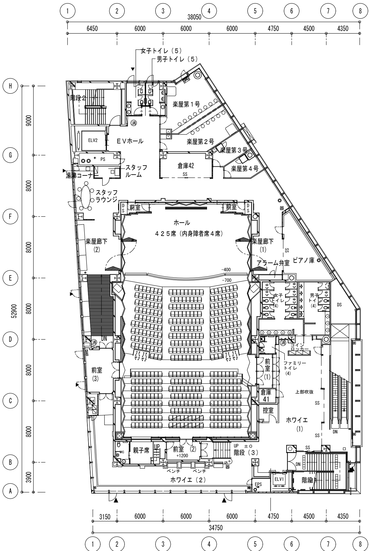
4階平面図 1/300
