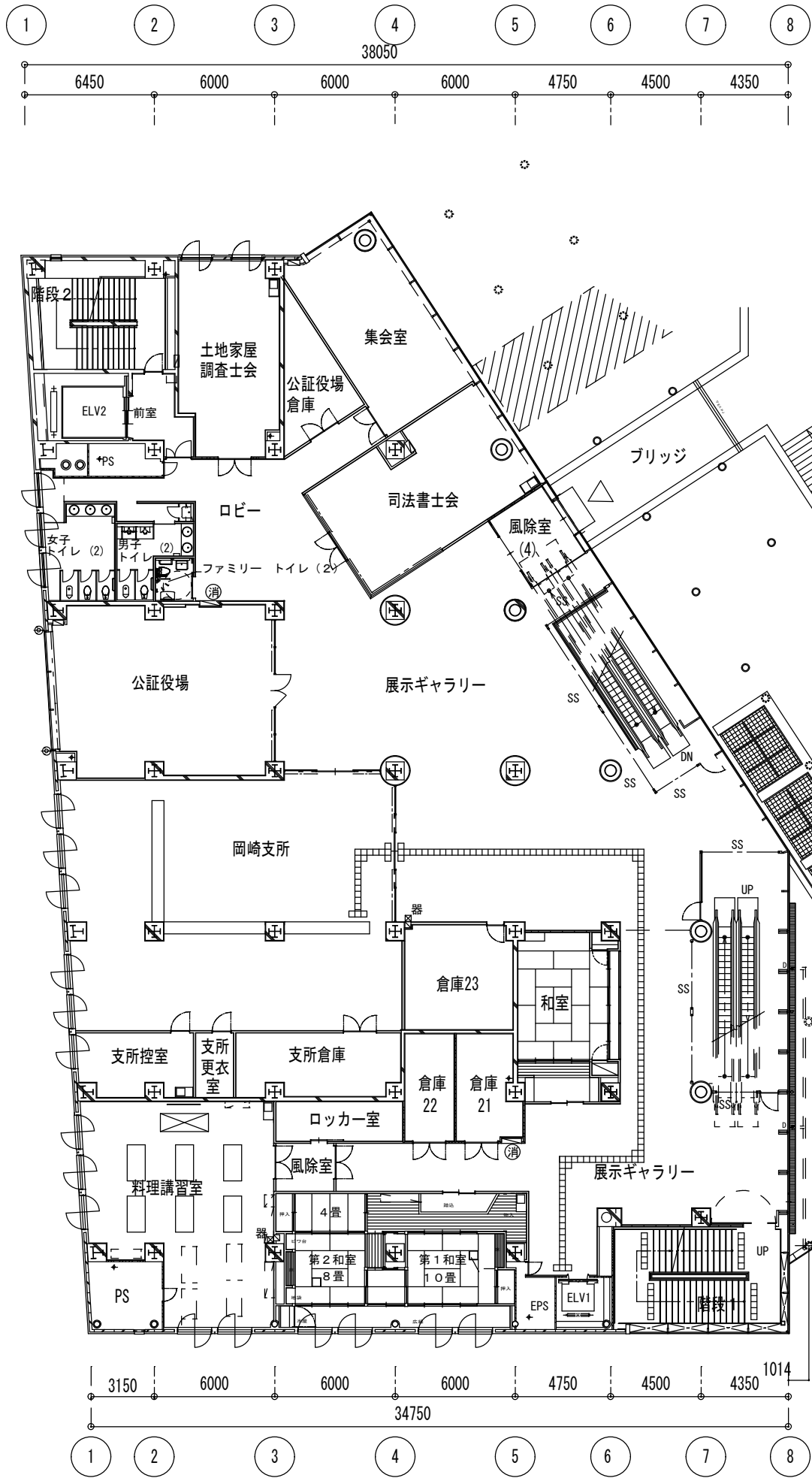
2階平面図 1/300
